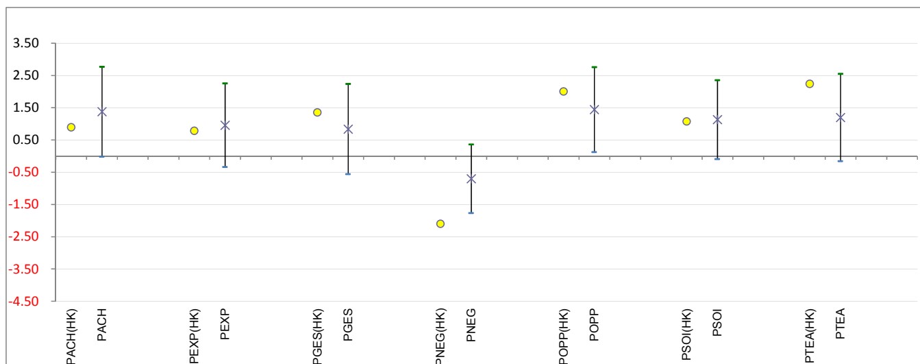
平均圖—原始分數—香港常模—全體報告
